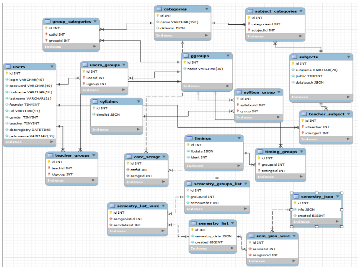
Рисунок 2. База данных
